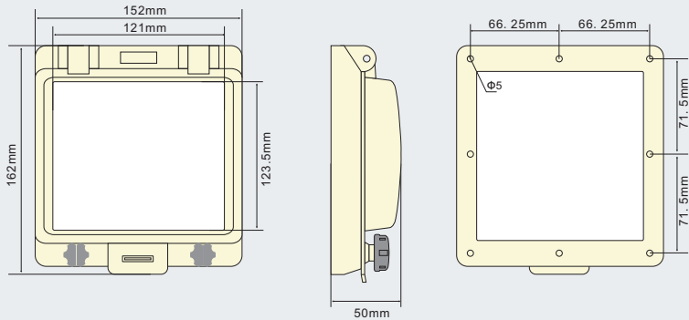
PWW-400K - Abmessungen und Montagebohrungen
