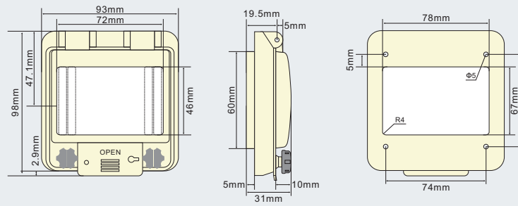
PWW-6 - Abmessungen und Montagebohrungen
