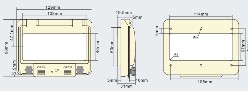
PWW-6 - Abmessungen und Montagebohrungen
