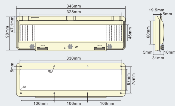
PWW-5 - Abmessungen und Montagebohrungen
