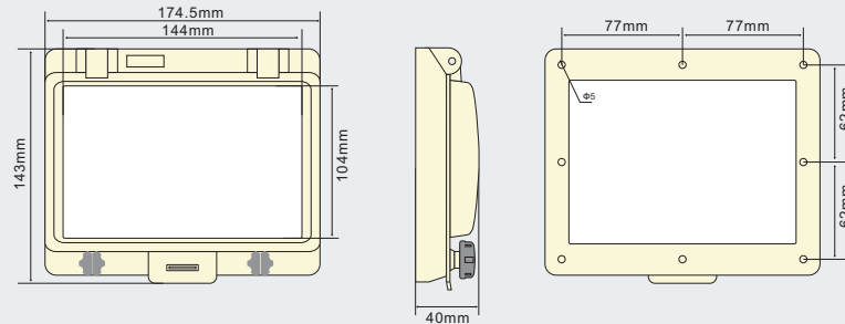
PWW-144K - Abmessungen und Montagebohrungen
