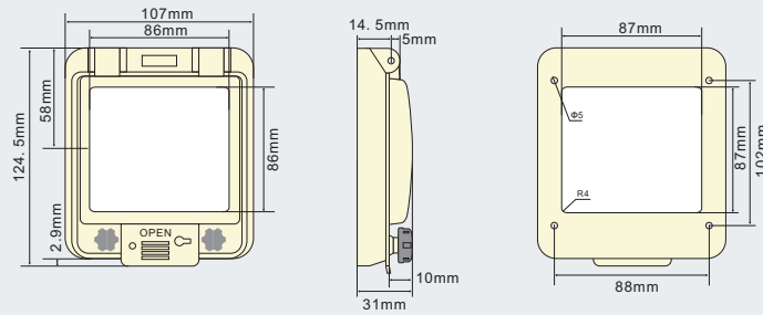
PWW-144K - Abmessungen und Montagebohrungen
